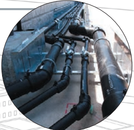
アイボリーブロードパイプ 融雪・消雪配管 施工現場
