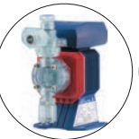
デジタルコントローラー搭載 フリー電源 電磁定量ポンプ (EHN)
